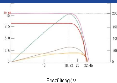
Áram-feszültség jellemzők
