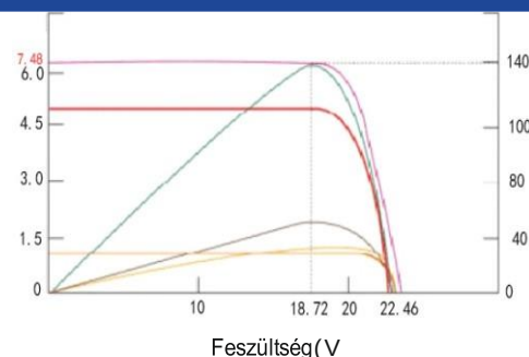
Áram-feszültség jellemzők
