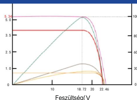
Áram-feszültség jellemzők
